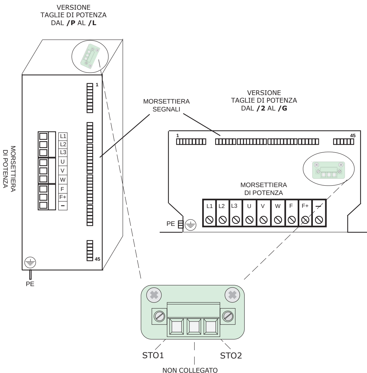
Fig.4: morsetti per la funzione STO sui pannelli moresettiere degli inverter.
